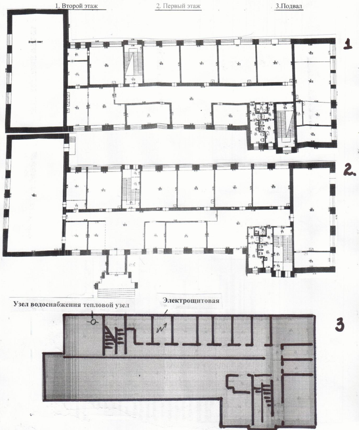
Поэтажный план (схема) объекта МБОУ «Елунинская ООШ» с обозначением критических элементов объектов
